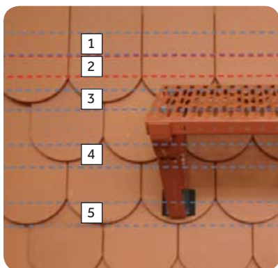
Obr. 10 - Popis k obrázku (vzdálenost latí je 145 mm) 1 - střešní latě, 2 - mezilatě, 3 - střešní latě, 4 - střešní latě, 5 - střešní latě
