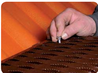
Obr. 6 Připevnění stoupací lávky
