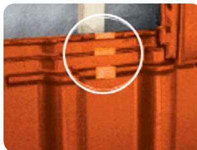
Obr. 8 Úprava drážky
