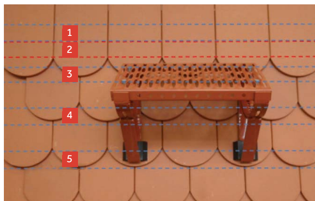
Obr. 9 - Popis k obrázku (vzdálenost late je 145 mm)
