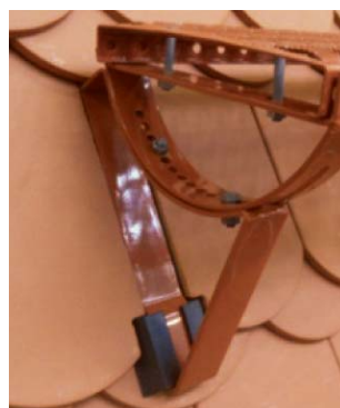
Obr. 10 – Popis k obrázku (vzdálenost latí je 290 mm) 1 - střešní lať, 2 - mezilať, 3 - střešní lať, 4 - střešní lať
